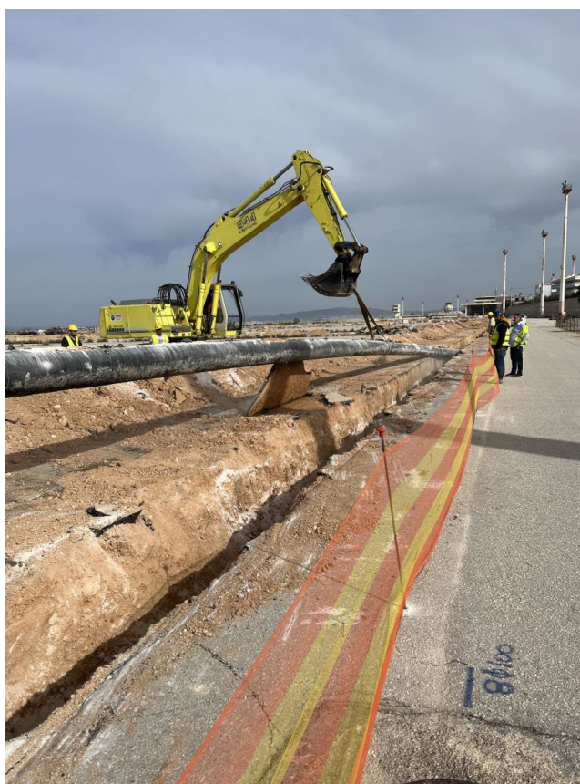
Εικόνα 5: Απομάκρυνση υπόγειου αγωγού καυσίμων
